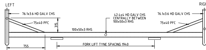
ELEVATION B 1:20
