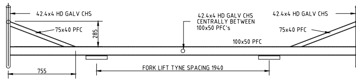
ELEVATION B 1:20
